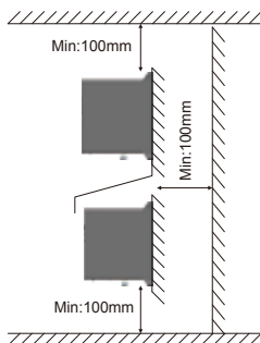
图3 上下安装
